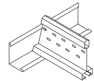
Querschiene zugeschnitten für Randwinkel
